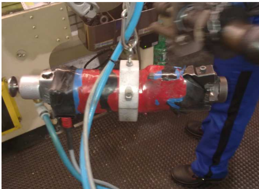
Pneumatické lisovacie kliešte YOKOTA typ YSA-4T-X48 v prevádzke
